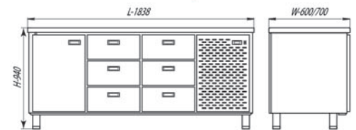
СШС-6,1-1850 / СШН-6,1-1850
