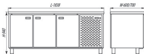
СШС-0,3-1850 / СШН-0,3-1850
