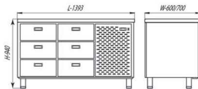
СШС-6,0-1400 / СШН-6,0-1400
