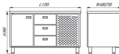
СШС-3,1-1400 / СШН-3,1-1400
