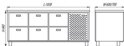
СШС-6,0-1850 / СШН-6,0-1850
