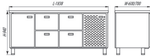
СШС-4,1-1850 / СШН-4,1-1850
