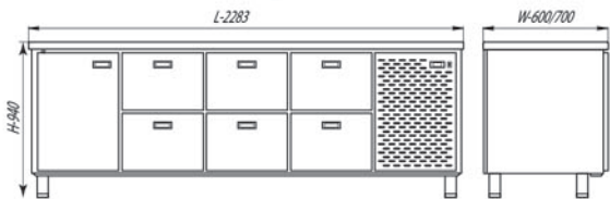
СШС-6,1-2300 / СШН-6,1-2300
