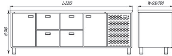
СШС-4,2-2300 / СШН-4,2-2300
