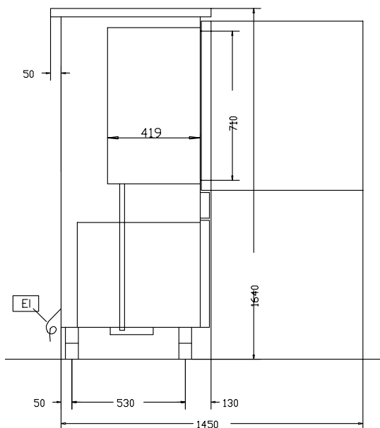
Вид сбоку
